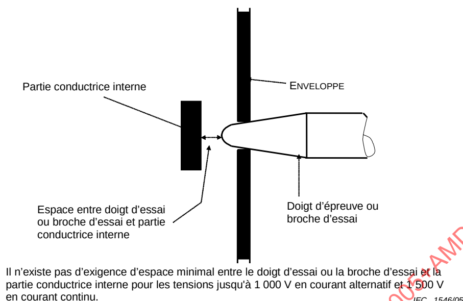
Figure 2D – Accessibilité des parties conductrices internes
