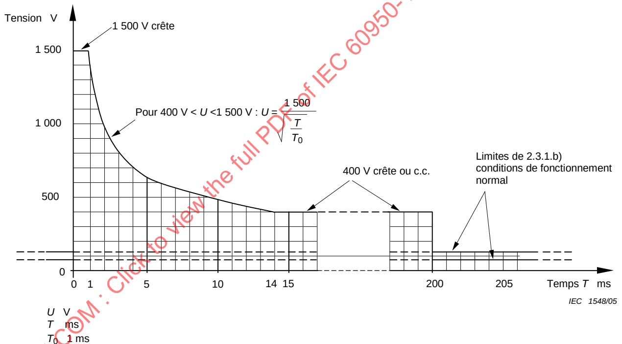
Figure 2F – Tensions maximales admises après un premier défaut
