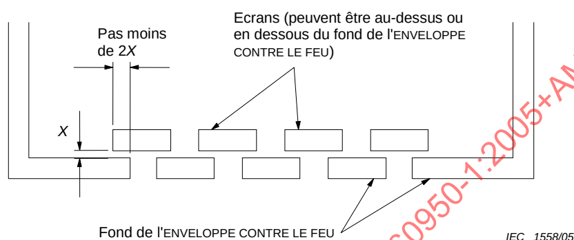
Figure 4F – Construction avec plaque écran
