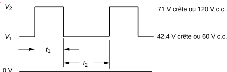
Figure 2E – Tensions dans les circuits TBTS dans les conditions de premier défaut
