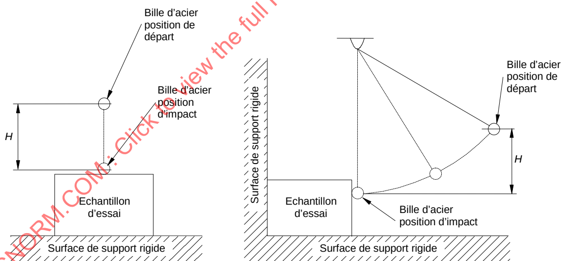
Figure 4A – Essai de choc utilisant la sphère d'acier
