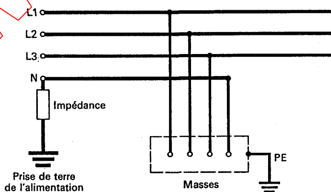
Figure 5 - Exemple de SCHÉMA D'ALIMENTATION IT
