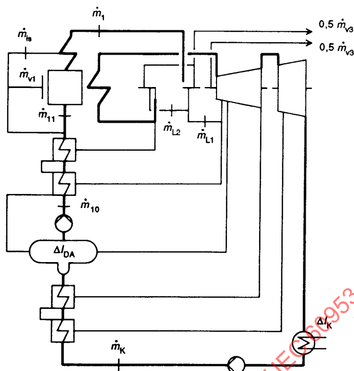
FIG. D1. — Schéma du cycle d'une centrale avec turbine à vapeur à simple resurchauffe et cinq soutirages pour réchauffage de l'eau d'alimentation.
