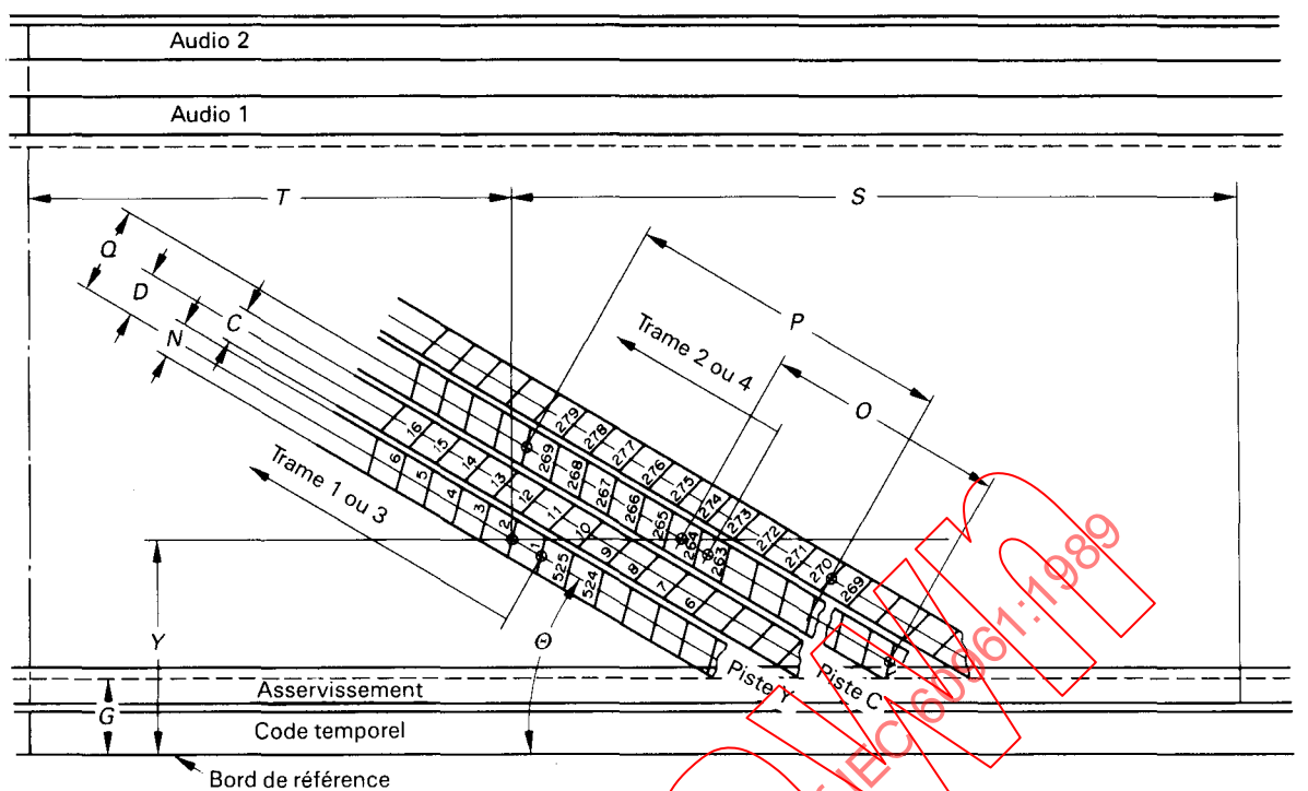
FIG. 4a. - Position des pistes enregistrées (525/60).
