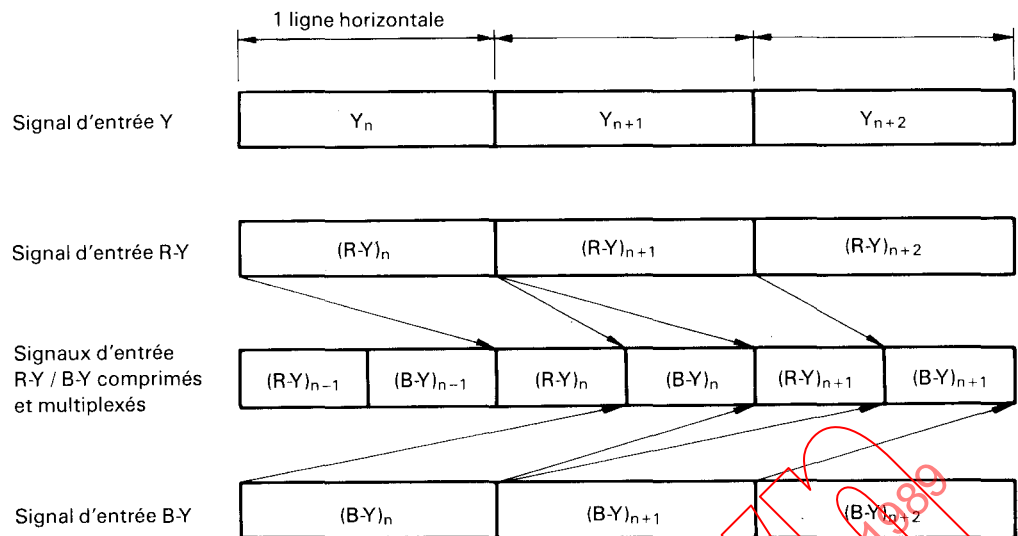
FIG. 8. – Système de compression et de multiplexage dans le temps.
