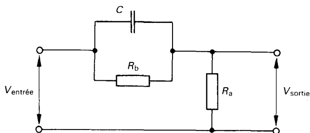
FIG. 6. - Réseau de préaccentuation.
