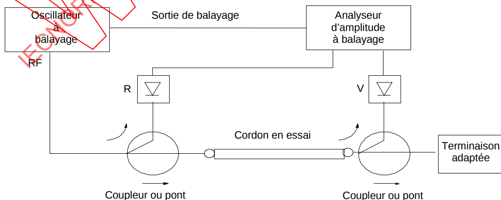
Figure A.3 – Circuit de remplacement permettant de déterminer les pertes d'insertion
