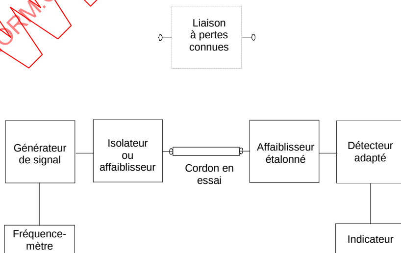
Figure A.1 – Circuit permettant de déterminer les pertes d'insertion
