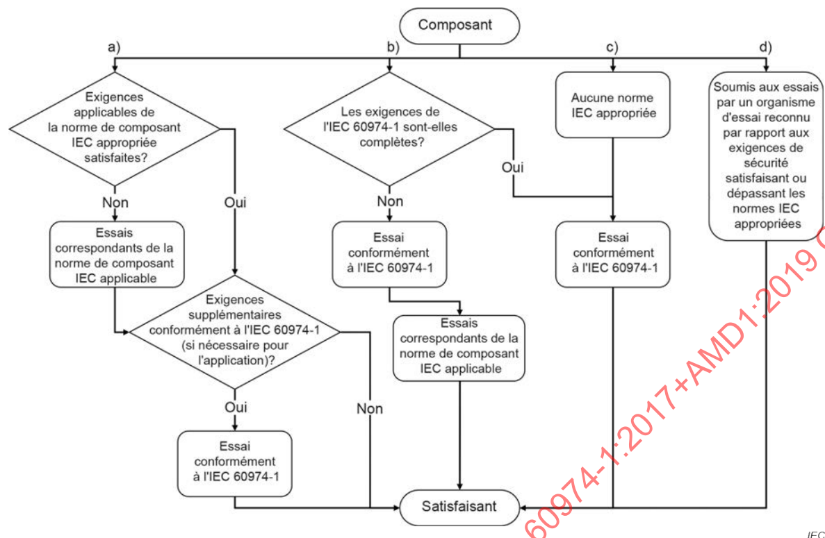
Figure P.1 – Diagramme pour les méthodes de conformité de l'Annexe P
