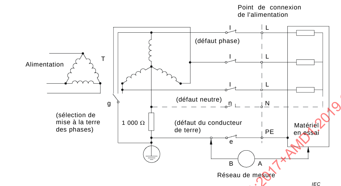
c) Matériel triphasé sur système IT en étoile
