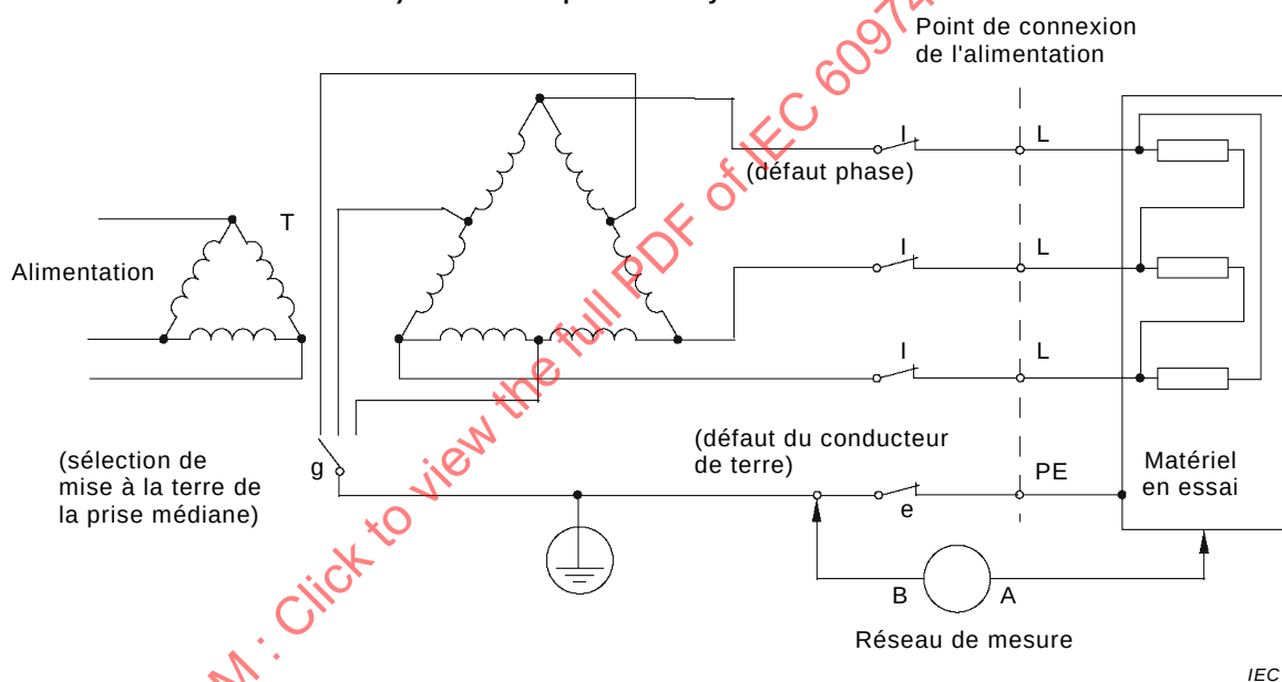
d) Matériel triphasé sur système triphasé à trois lignes centré et relié à la terre
