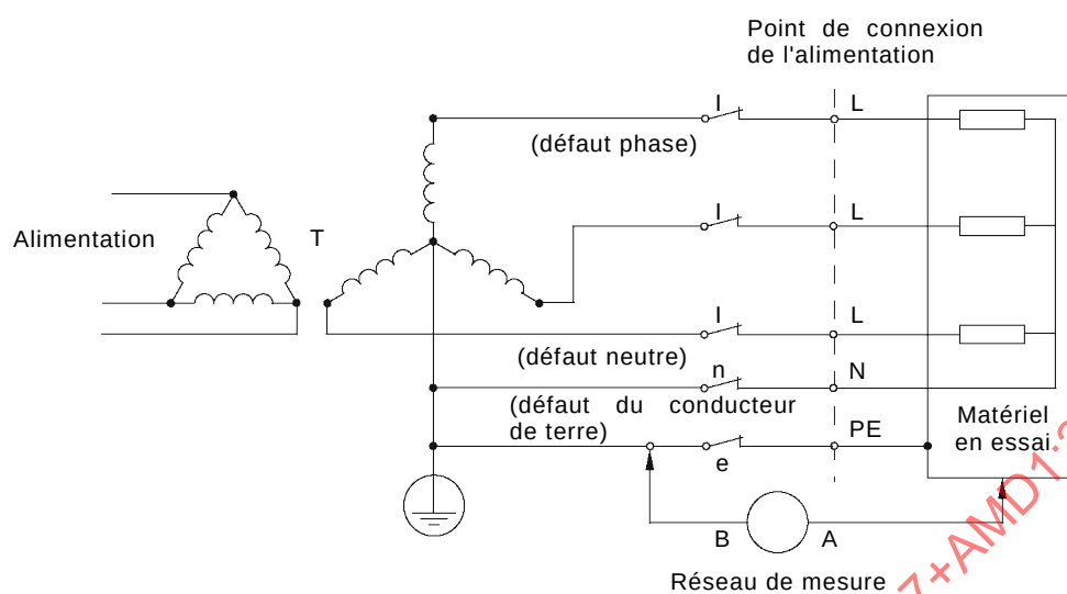
a) Matériel triphasé sur système TT ou TN en étoile
