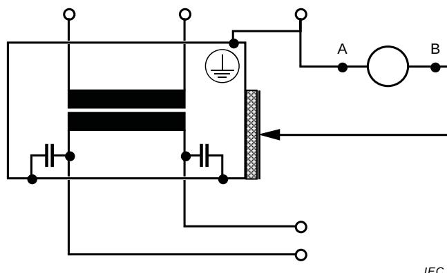
Figure 3 – Mesurage du courant de contact en condition normale
