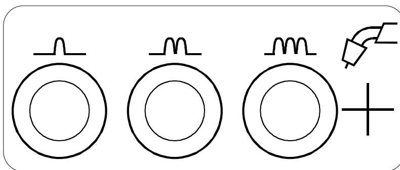
Figure L.4 – Bornes avec sélecteurs d'inductance pour le soudage MIG/MAG
