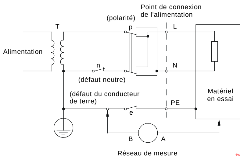
a) Matériel monophasé sur un système TT ou TN en étoile
