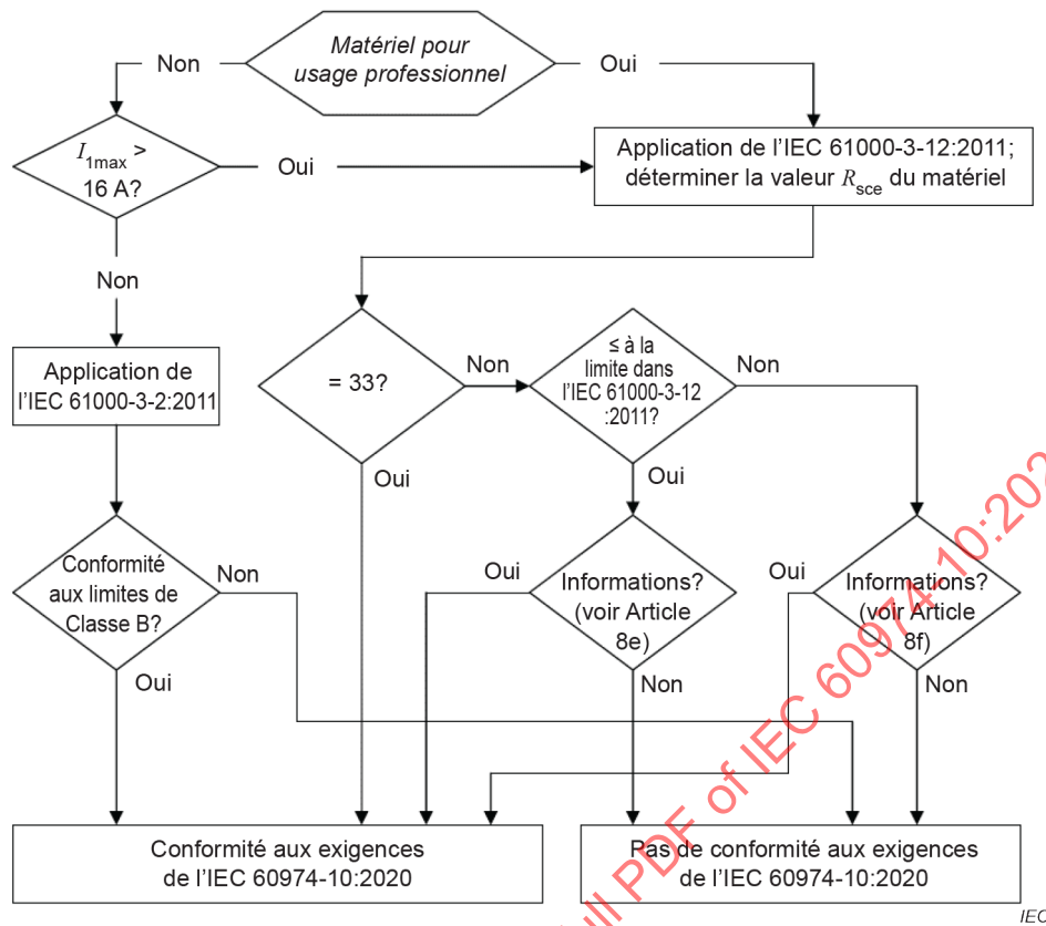
Figure 5 – Présentation des exigences concernant les harmoniques pour un courant d'alimentation I_{1\max} allant jusqu'à 75 A
