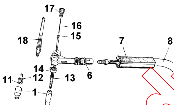
Figure A.3 – Torche pour soudage à l'arc en atmosphère inerte avec électrode de tungstène
