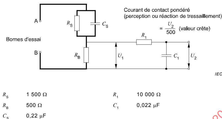
Figure 4 – Réseau de mesure, courant de contact pondéré pour la perception ou la réaction de tressaillement
