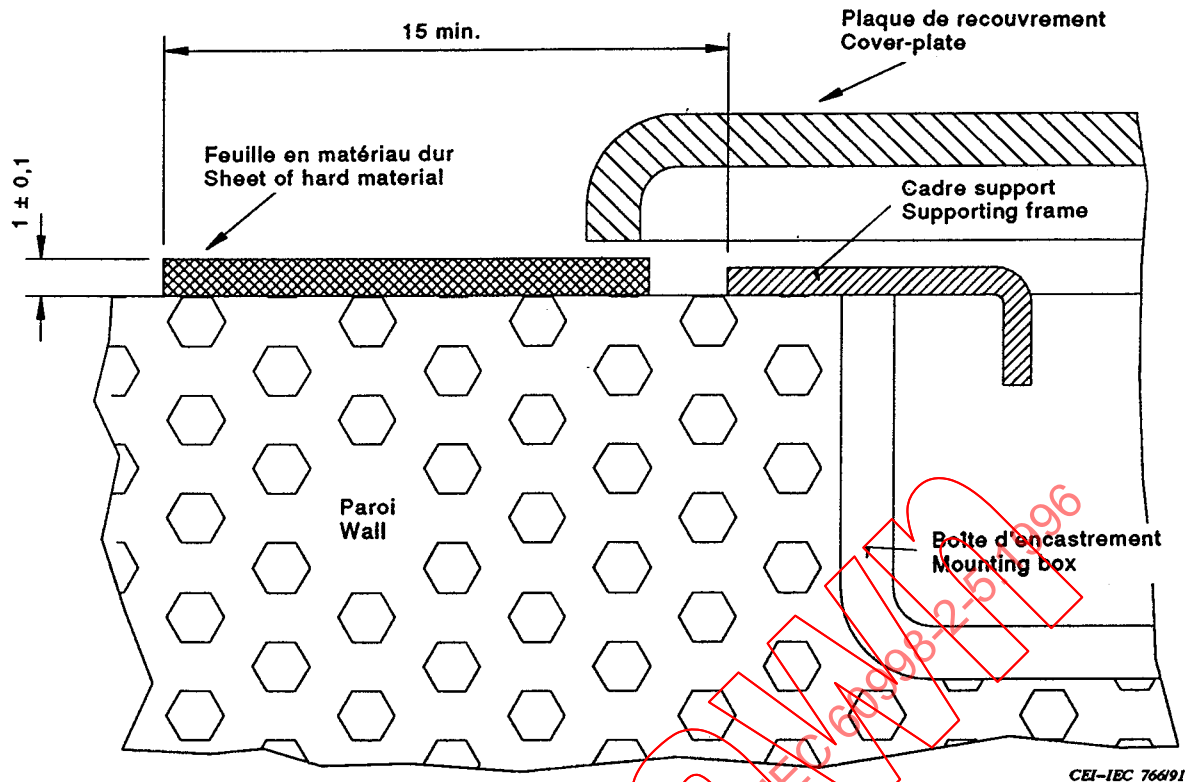
Figure 101 – Disposition pour l'essai des plaques de recouvrement Arrangement for test on cover-plates
