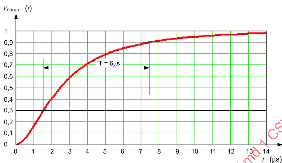
Figure E.8 – Tension de choc (10/700 \mu\text{s} ): réponse de temps de montée T
