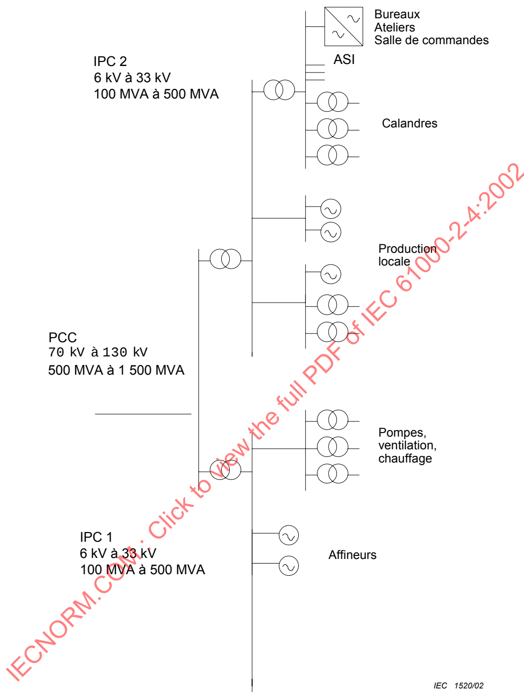
Figure B.2 – Exemple de distribution de puissance dans l'industrie papetière
