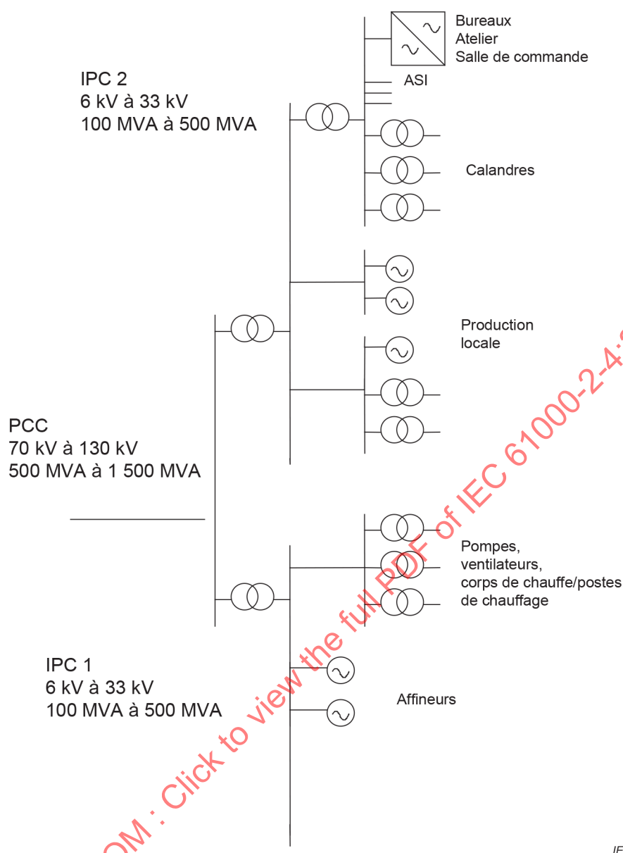
Figure B.2 – Exemple de distribution d'électricité dans l'industrie papetière
