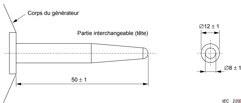
3a) – Electrode de décharge pour les décharges dans l'air
