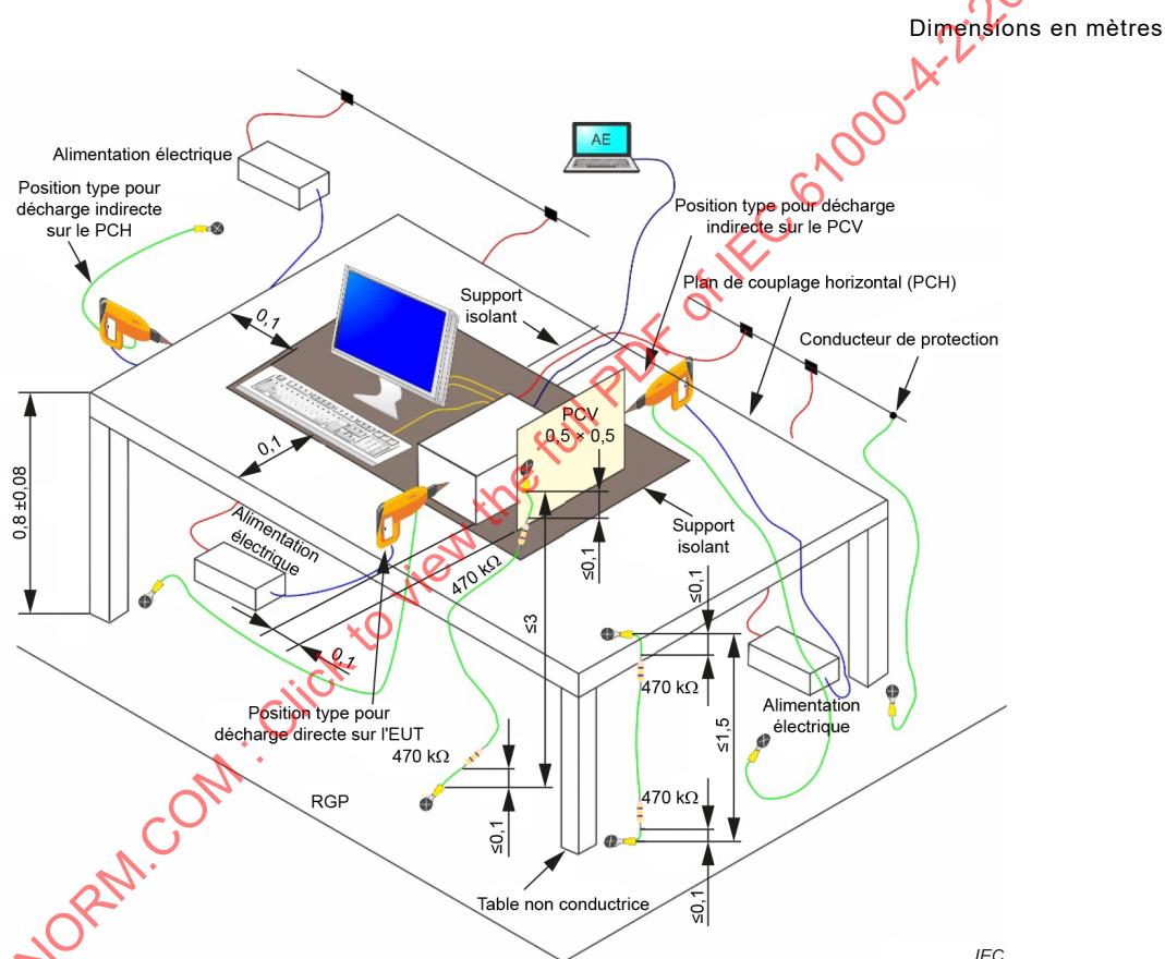
Figure 6 – Exemple de montage d'essai pour un matériel de table
