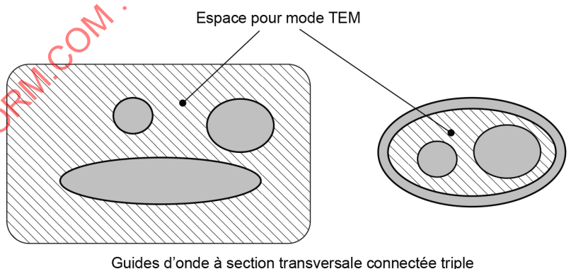
Figure D.2 – Exemple de guides d'onde prenant en charge la propagation en mode TEM (voir D.3.3)
