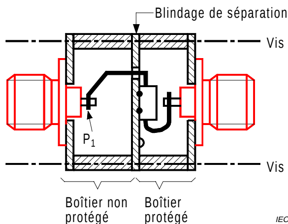
Figure 3 – Exemple de dispositif d'essai de type B à quatre accès dans une configuration sans passe-paroi
