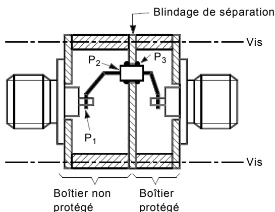
c) Exemple de dispositif/support d'essai comportant un DUT au sein d'une configuration avec traversée
