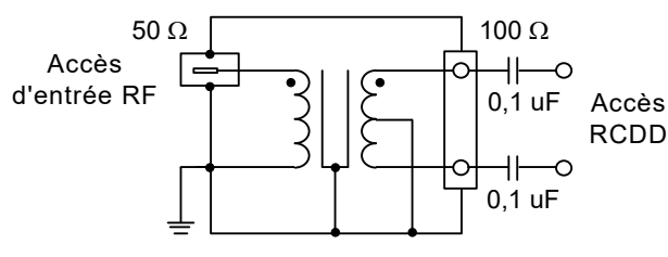
Figure 7 – Schéma de circuit type du montage de transformateur représentant les côtés 50 Ω et 100 Ω du transformateur et 2 éléments de condensateurs de couplage de 0,1 μF
