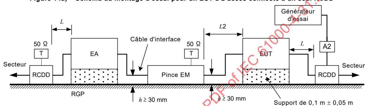
Figure 14b) – Schéma du montage d'essai lorsque l'EA présente des erreurs au cours de l'essai
