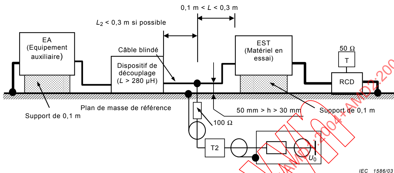
Figure 5b – Principe de l'injection directe sur câbles blindés
