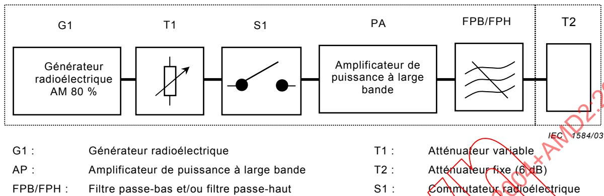
Figure 3 – Montage du générateur d'essai
