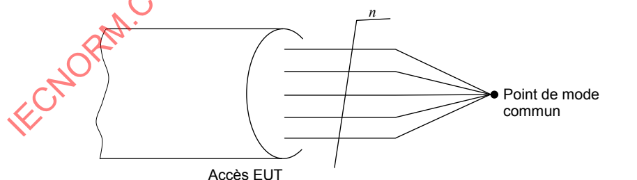
a) Définition d'un point de mode commun avec câbles non blindés
