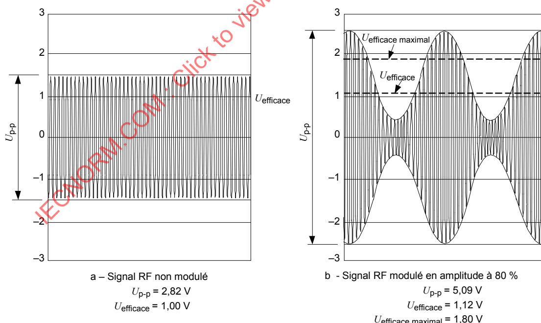
Figure 2 – Formes d'onde en circuit ouvert se produisant à l'accès EUT d'un dispositif de couplage pour le niveau d'essai 1
