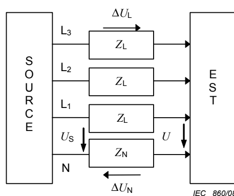
Figure 3 – Montage pour la mesure des émissions triphasées
