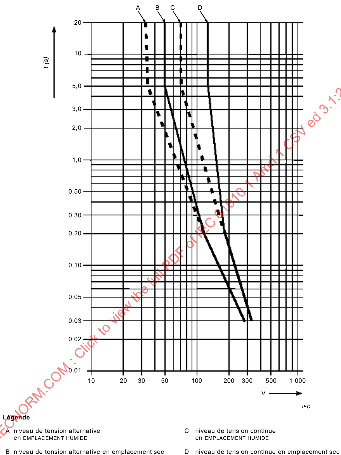
Figure 2 – Durée maximale des tensions de courte durée accessibles en CONDITION DE PREMIER DEFAT (voir 6.3.2 a))
