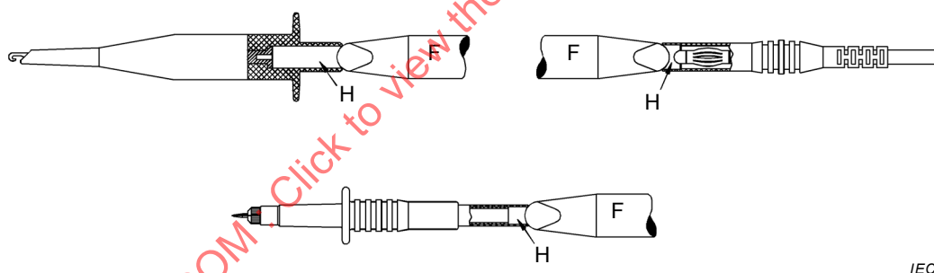
Figure 6c – Sonde équipée partiellement couplée (voir 6.2 et 6.4.2b))
