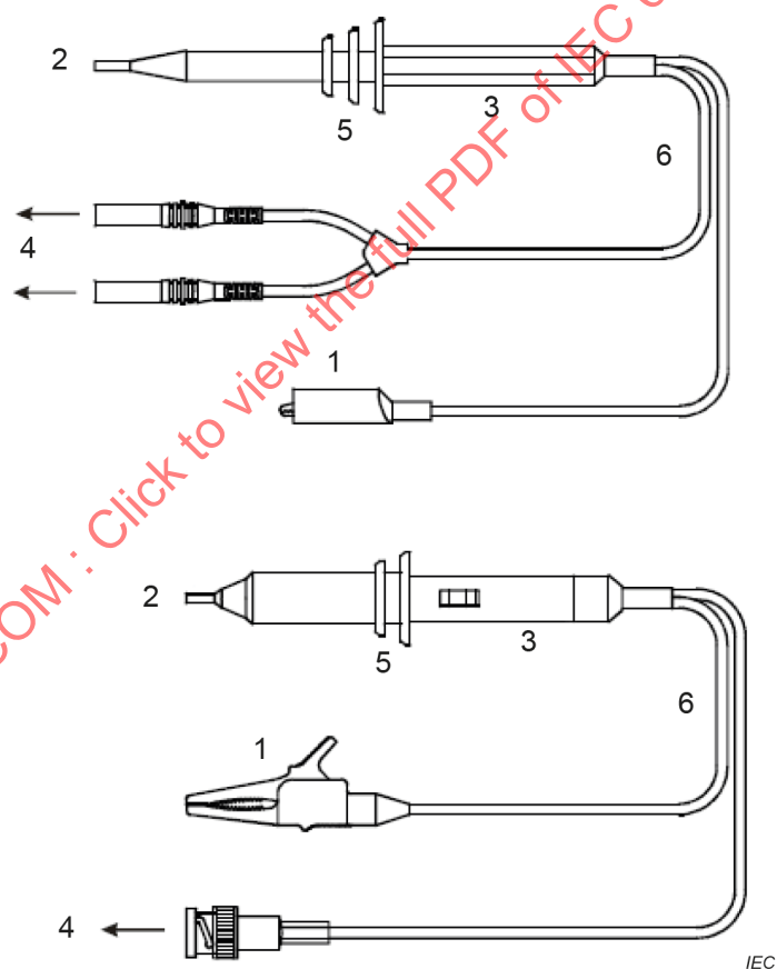
Figure 2 – Exemples de sondes équipées de type A
