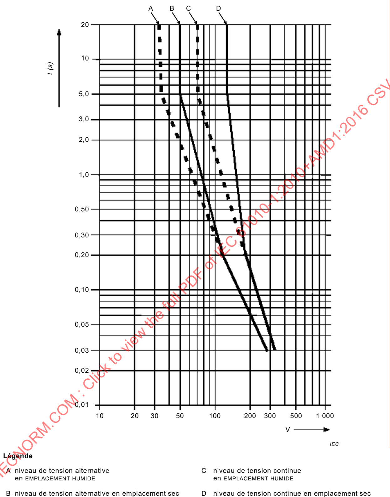
Figure 2 – Durée maximale des tensions de courte durée accessibles en CONDITION DE PREMIER DEFAT (voir 6.3.2 a))
