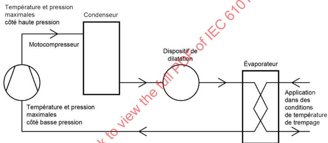
Figure 101 – Schéma d'un système frigorifique comportant un condenseur
