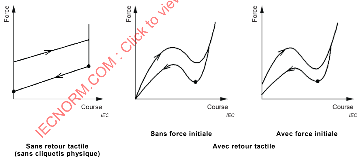
Figure 2 – Exemple de points de mesure stipulés dans les spécifications particulières
