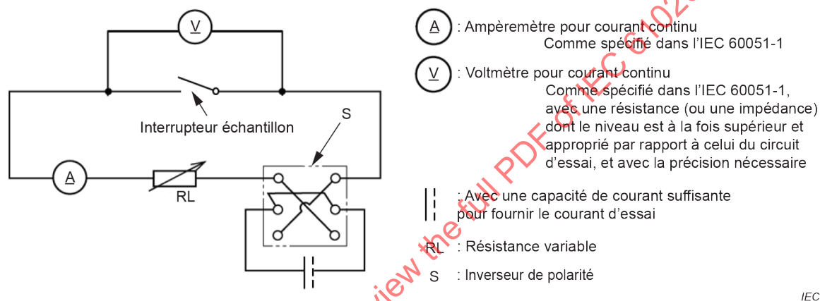
Figure 7 – Méthode à courant spécifié (en courant continu)
