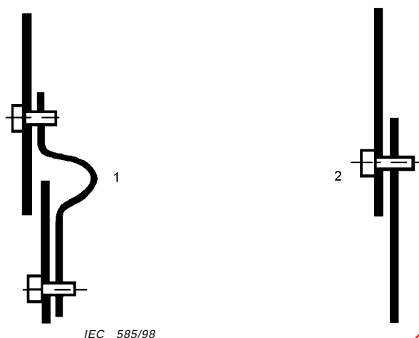
1 Pontage métallique souple
