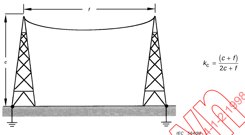
Figure 32 – Valeurs du coefficient k_c dans le cas d'un dispositif de capture aérien et d'une prise de terre de type A
