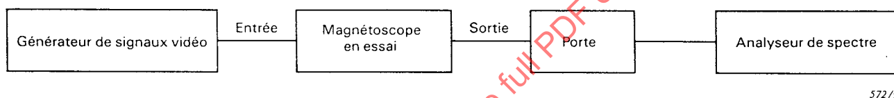
Figure 13 - Circuit de mesure de l'intermodulation entre les voies chrominance et luminance (article 3.3)
