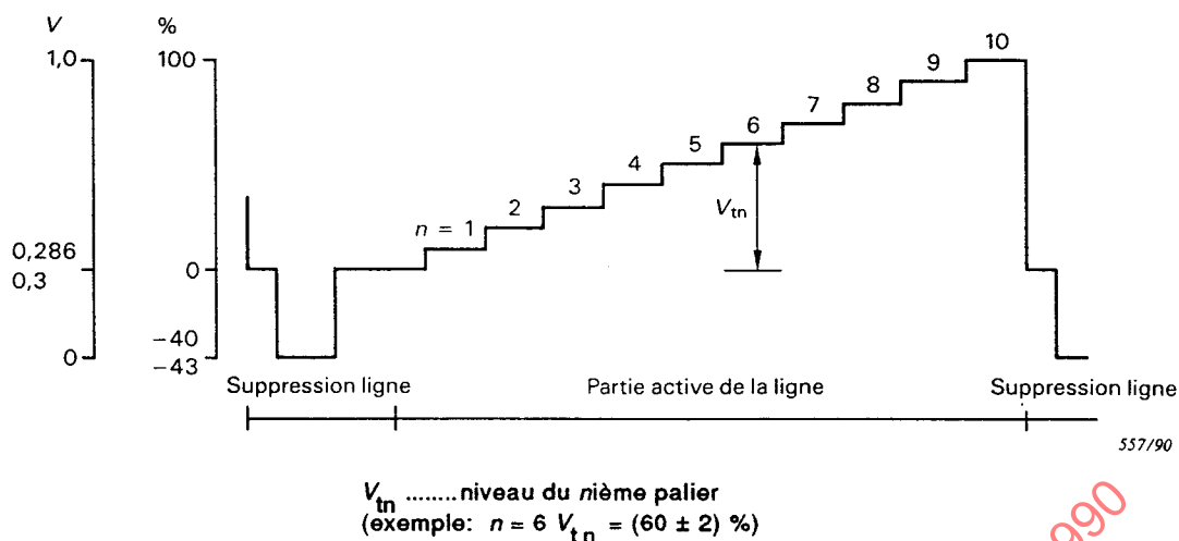
Figure 5 - Signal d'essai pour la mesure des distorsions non linéaires de la voie luminance (10 paliers) (article 2.4)
