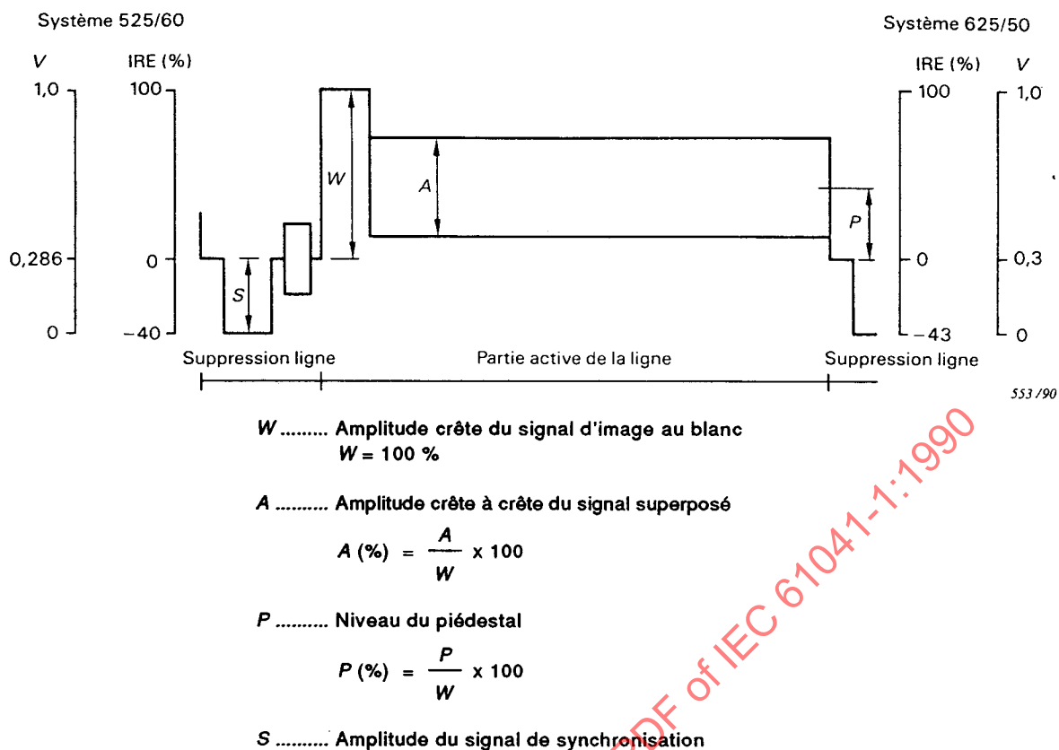
Figure 1 - Signal vidéo d'essai: valeurs nominales en ligne
