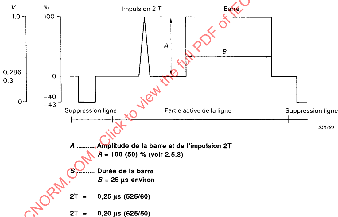
Figure 6 - Signal d'essai pour la mesure des distorsions linéaires sur les transitoires dans la voie luminance (article 2.5)
