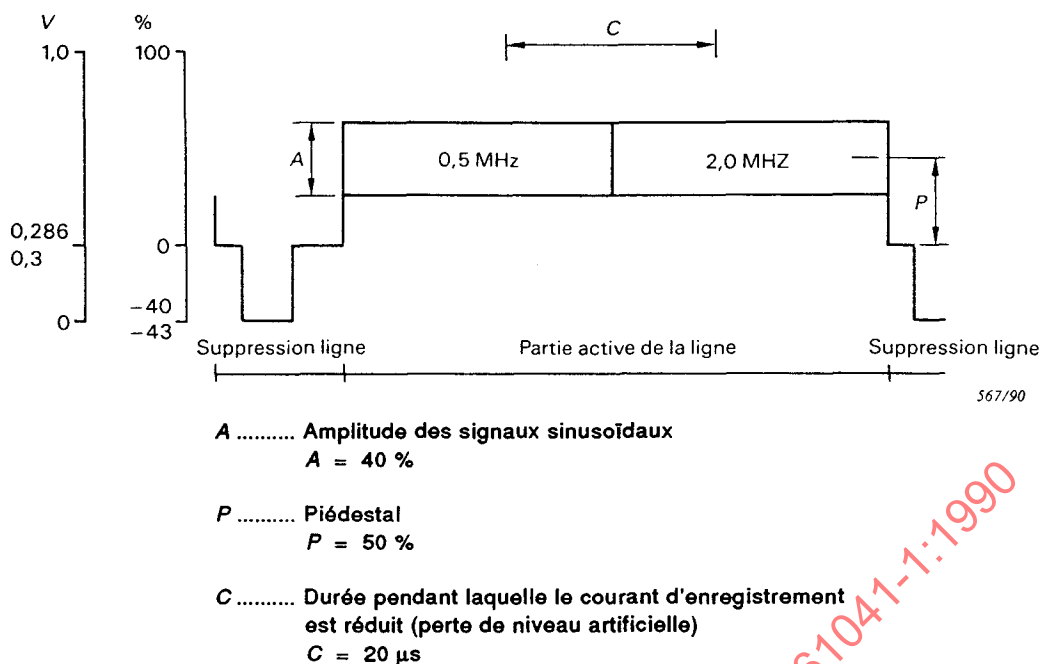
Figure 11b - Signal d'essai pour la mesure de la compensation des pertes de niveau luminance (préenregistré sur une bande d'essai)
