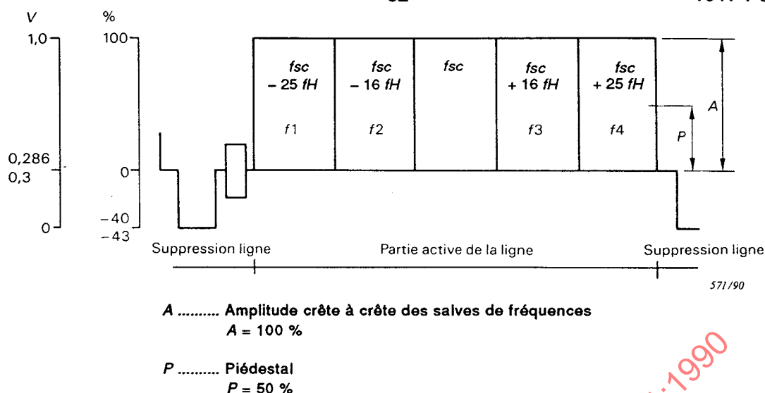
Figure 12 - Signal d'essai pour la mesure de la réponse amplitude/fréquence de la voie chrominance
