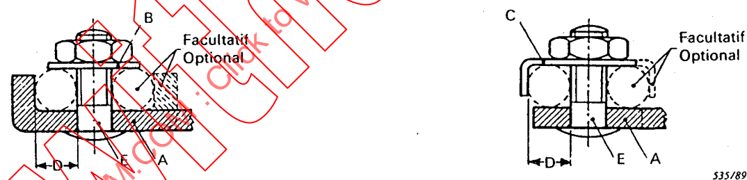
2b - Bornes à goujon fileté Stud terminals
