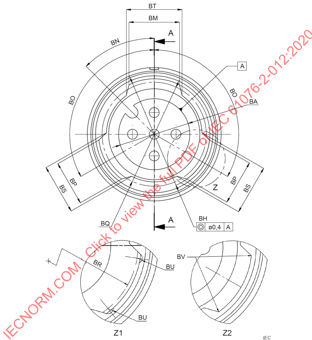
Figure 21 – Vue de face du côté femelle du boîtier de type pousser-tirer avec l'exemple d'un connecteur codé A
