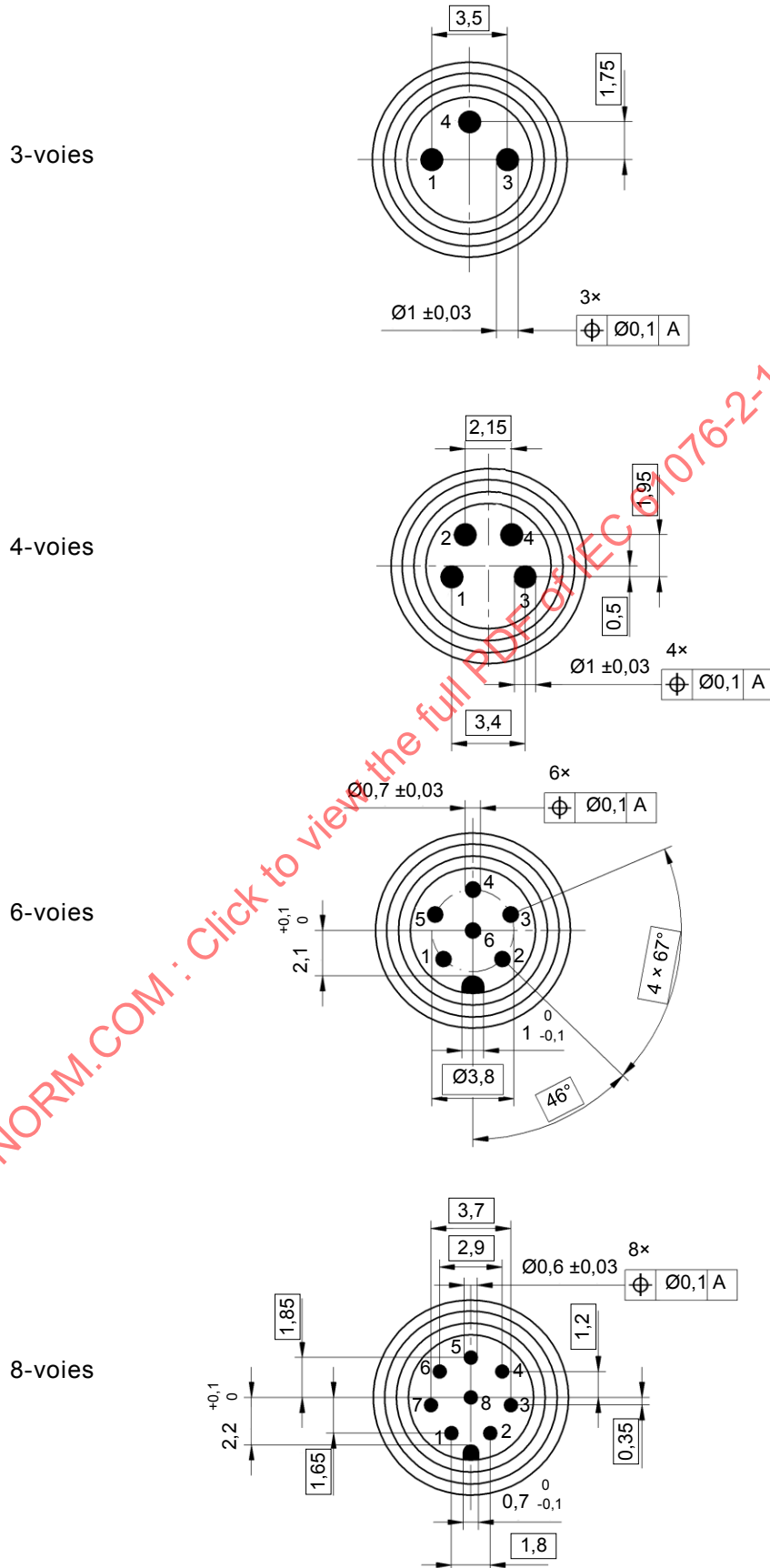
Figure 16 – Vue de face du contact mâle codage A
