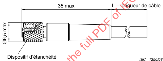
Figure 8 – Fiche non-démontable, contacts femelles, version à sortie droite, avec écrou de verrouillage
