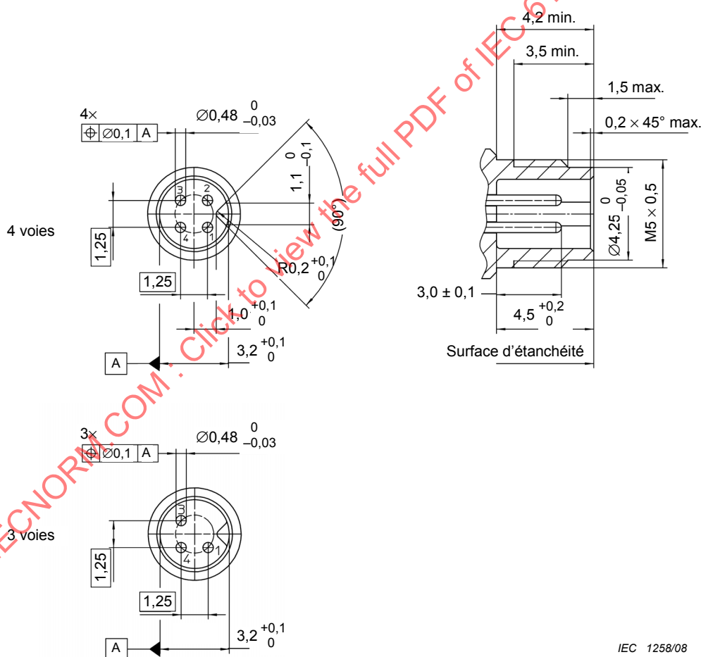
Figure 10 – Vue de face du contact mâle
