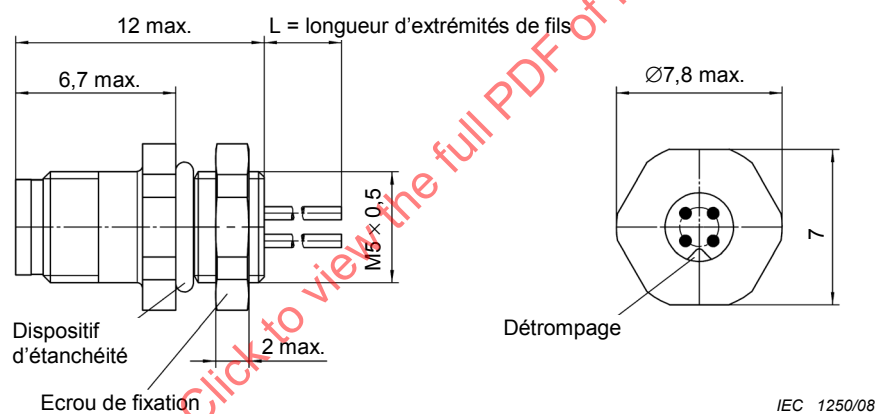
Figure 2 – Embase, contacts mâles, montage avec filet M5 x 0,5, avec extrémités de fils, montage par écrou M5 x 0,5, orientation du montage
