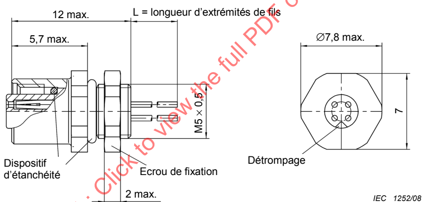
Figure 4 – Embase, contacts femelles, montage avec filet M5 × 0,5, avec extrémités de fils, montage par écrou, filet M5 × 0,5, orientation du montage
