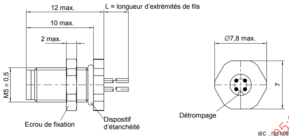
Figure 3 – Embase, contacts mâles, montage avec filet M5 × 0,5, avec extrémités de fils, montage arrière par écrou, filet M5 × 0,5, orientation du montage
