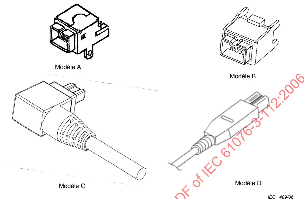
Figure 3 – Vue isométrique
