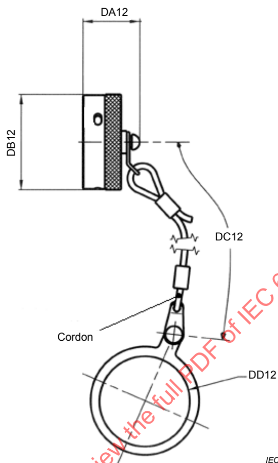
Figure 4 – Bouchon pour embase, variante 11
