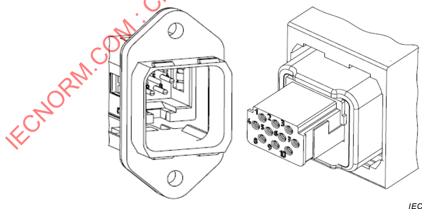
Figure 1 – Embases (mâles) et fiches (femelles)
