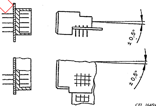
Figure 10 – Inclinaison
