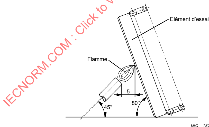
Figure 35 – Disposition pour l'essai d'inflammabilité
