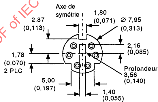
Figure 3d – Face d'accouplement à six positions
