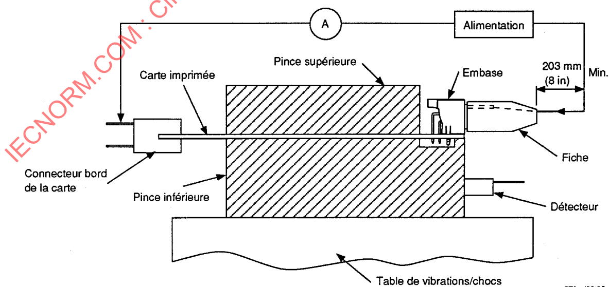
Figure 23 – Dispositif pour essai de contraintes dynamiques
