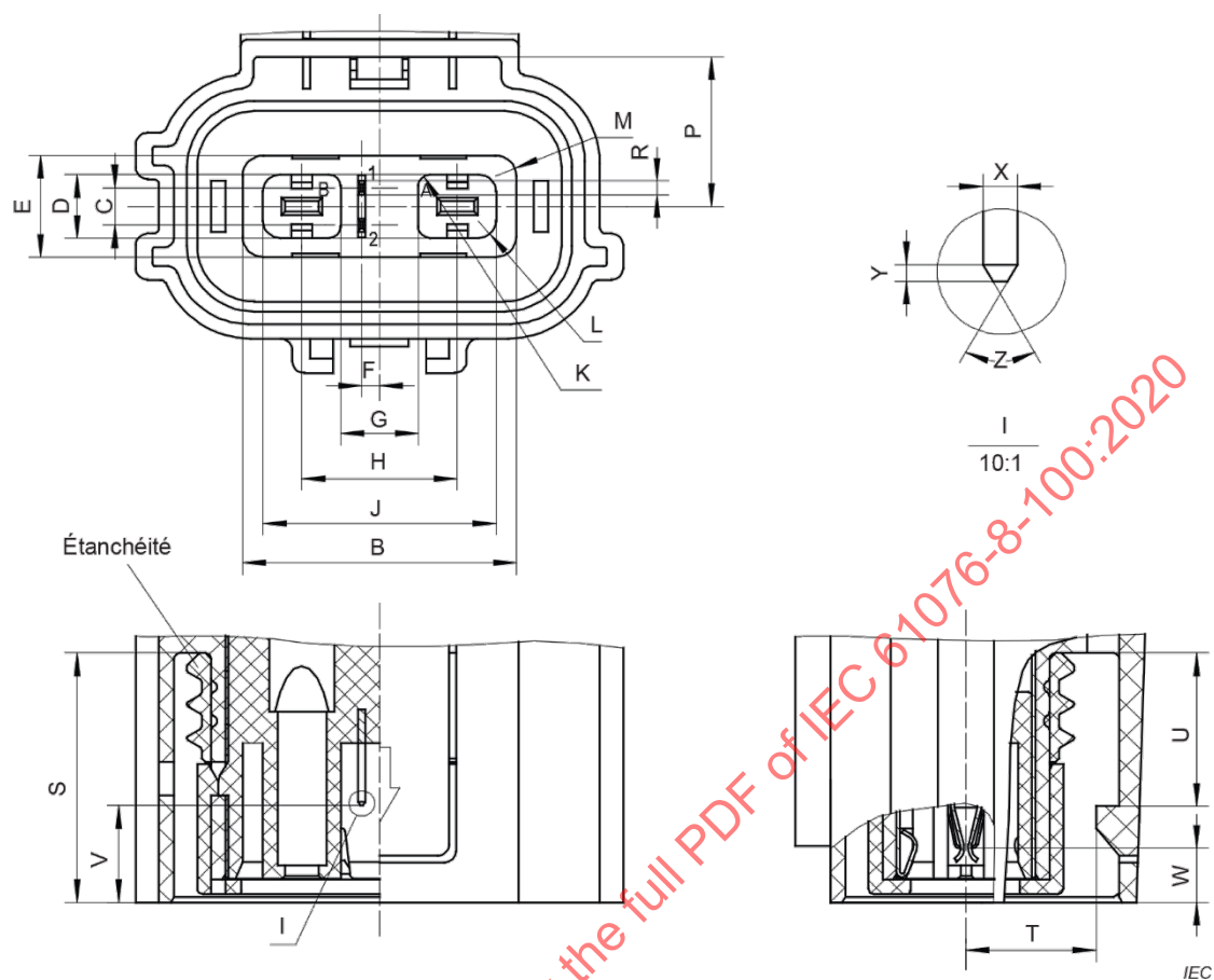
Figure 6 – Fiche bipolaire 20 A
