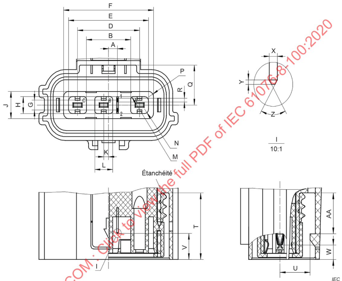
Figure 7 – Fiche tripolaire 20 A
