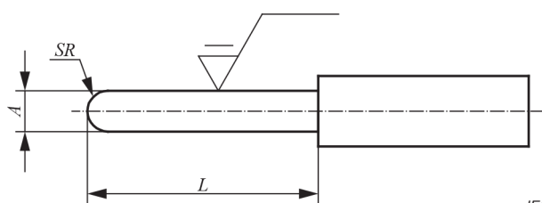
Figure 5 – Calibre pour contact
