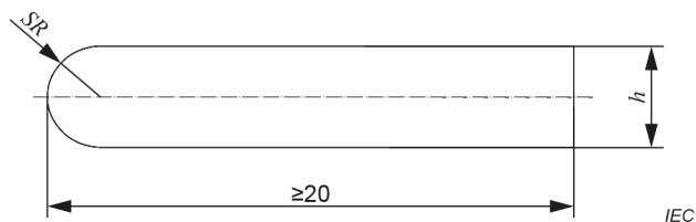
Figure 8 – Calibre pour contacts d'alimentation
