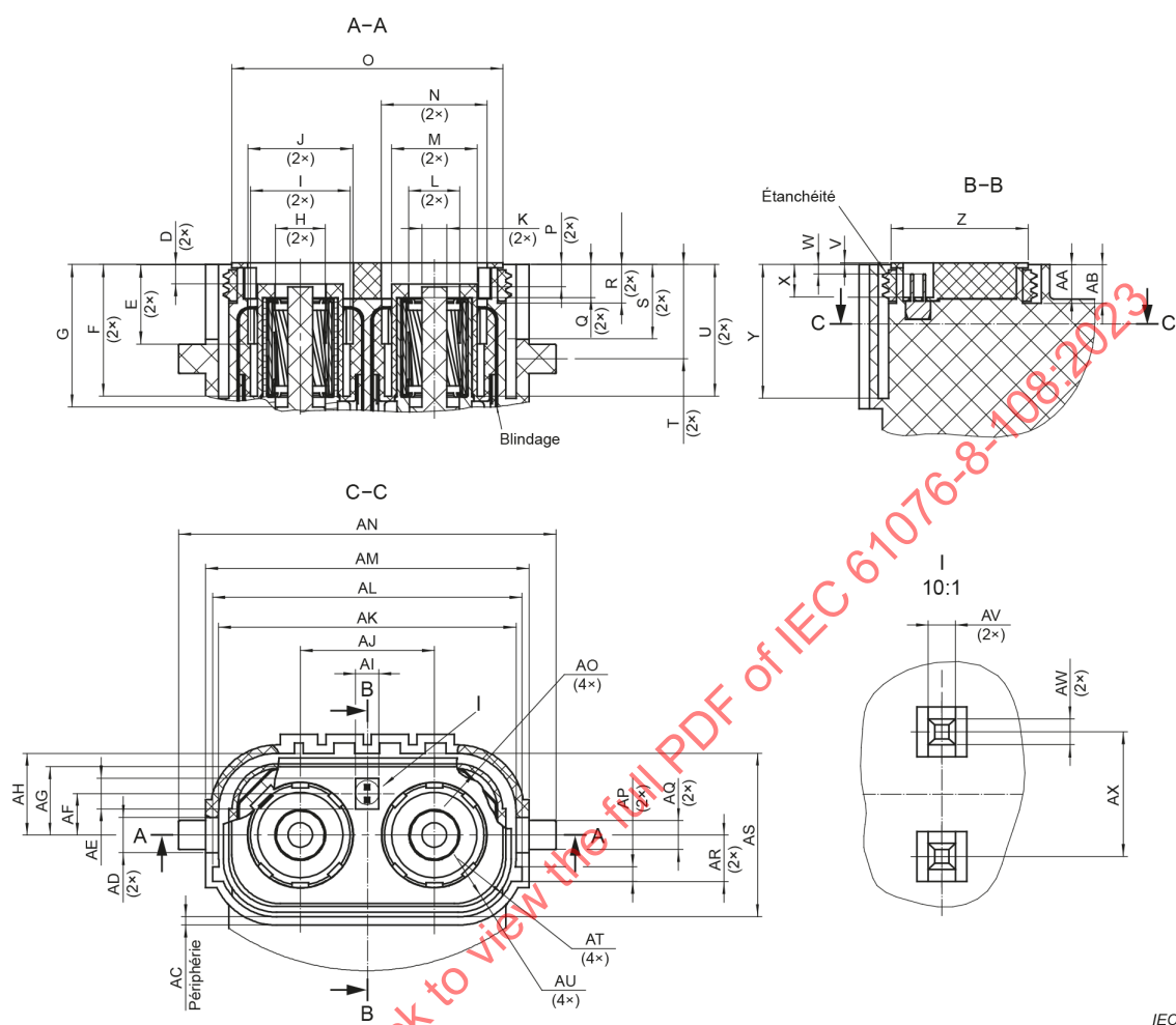
Figure 3 – Fiche
