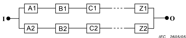
Figure 2 – Bloc-diagramme de fiabilité en séries dupliquées (ou parallèles)
