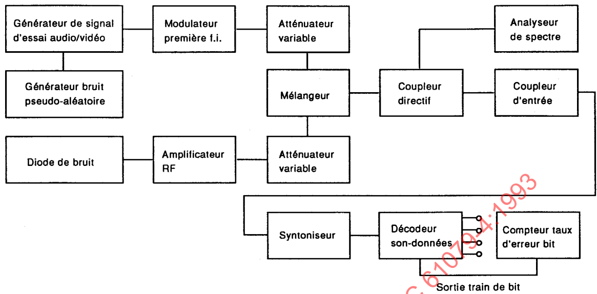
Figure 3 – Montage de mesure du taux d'erreur bit
