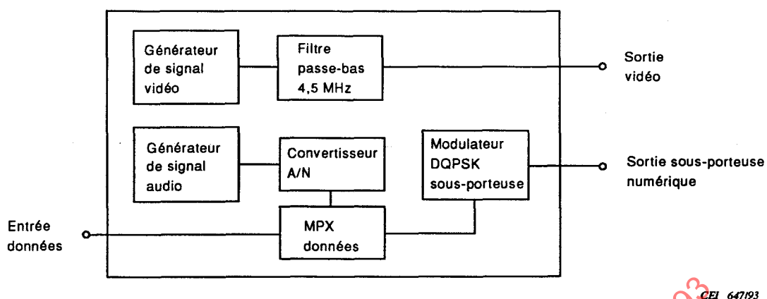
Figure 2a – Générateur de signal d'essai audio/vidéo
