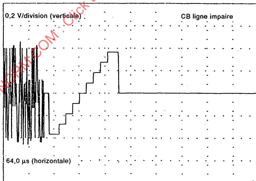
Figure 2g'' – Signal chrominance en escalier à huit fronts montants (ligne impaire)
