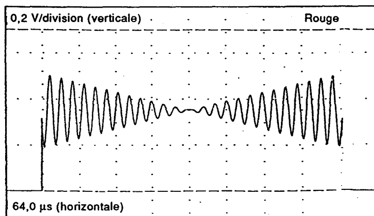
Figure 2j'' – Signal décodé couleur R résultant
