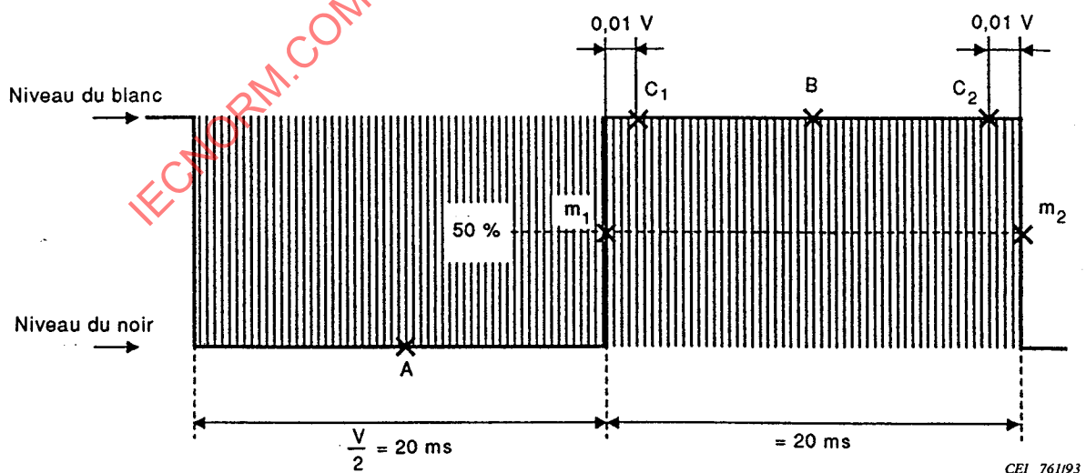
Figure 11 – Mesure des distorsions basse fréquence
