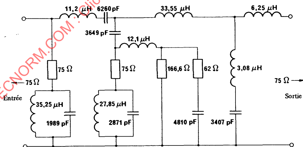
Figure 13 – Exemple de filtre de différentiation
