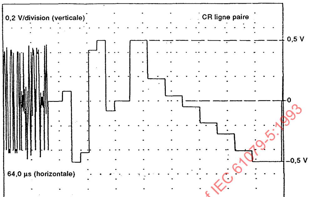
Figure 2i – Signal de barres de couleur 75 % (ligne paire)
