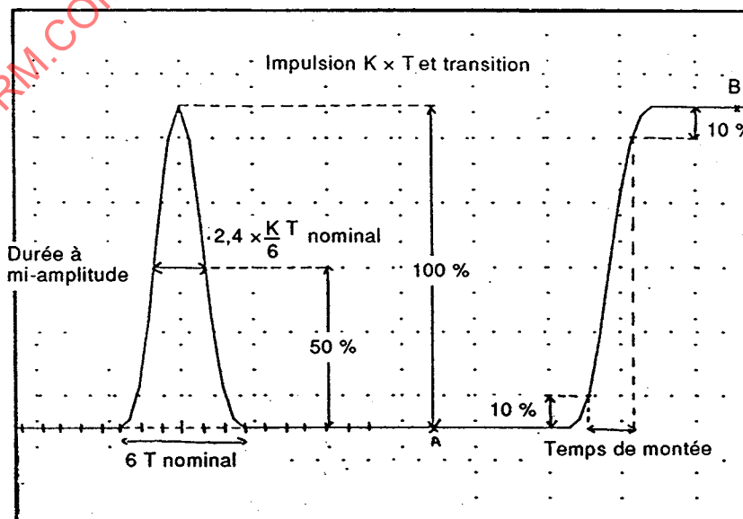
Figure 9 – Mesures de la réponse impulsionnelle et aux transitions
