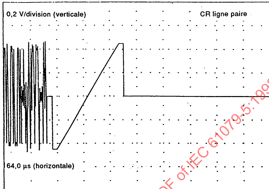
Figure 2f – Signal chrominance de rampe montante (ligne paire)
