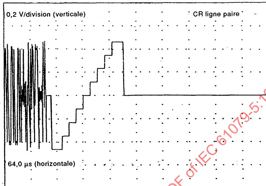
Figure 2g' – Signal chrominance en escalier à huit fronts montants (ligne paire)
