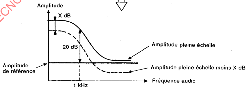
Figure 4 – Définition de l'amplitude de référence et de l'amplitude de pleine échelle
