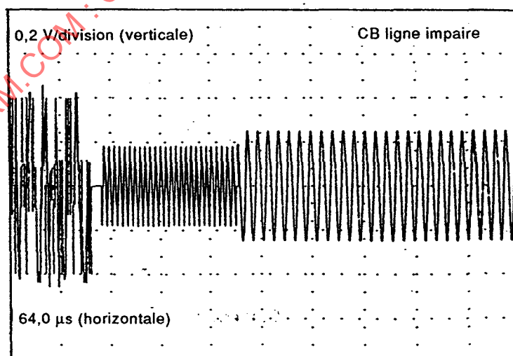
Figure 2j' – Signal d'essai noeud papillon (ligne impaire)
