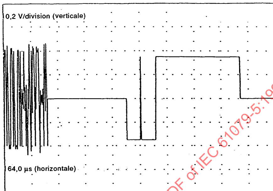
Figure 2e – Signal luminance d'impulsion et de barre
