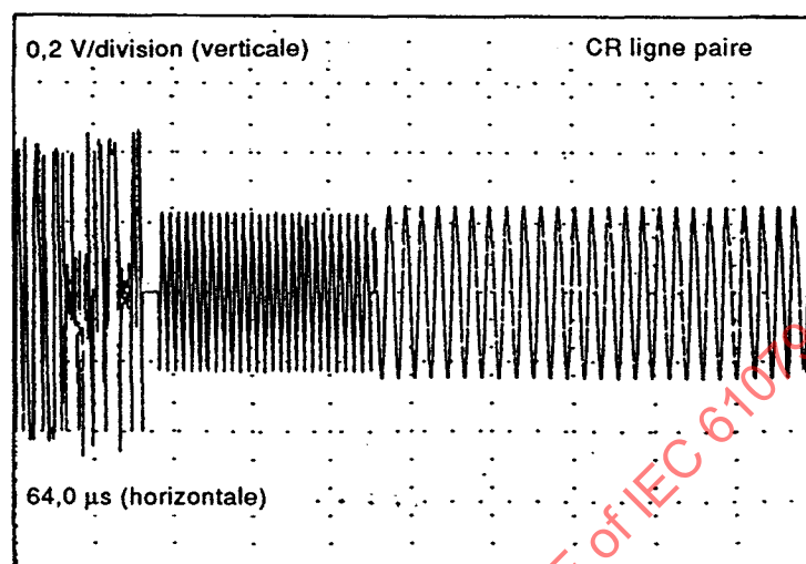
Figure 2j – Signal d'essai noeud papillon (ligne paire)
