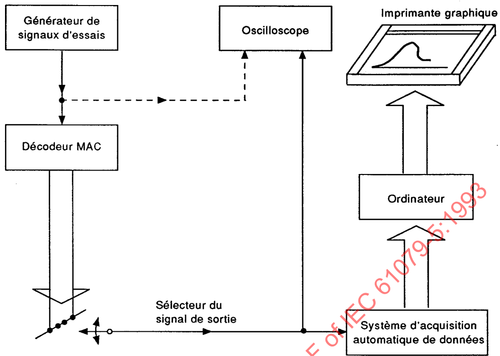
Figure 8 – Disposition des appareils pour l'acquisition et le calcul pour les mesures automatiques
