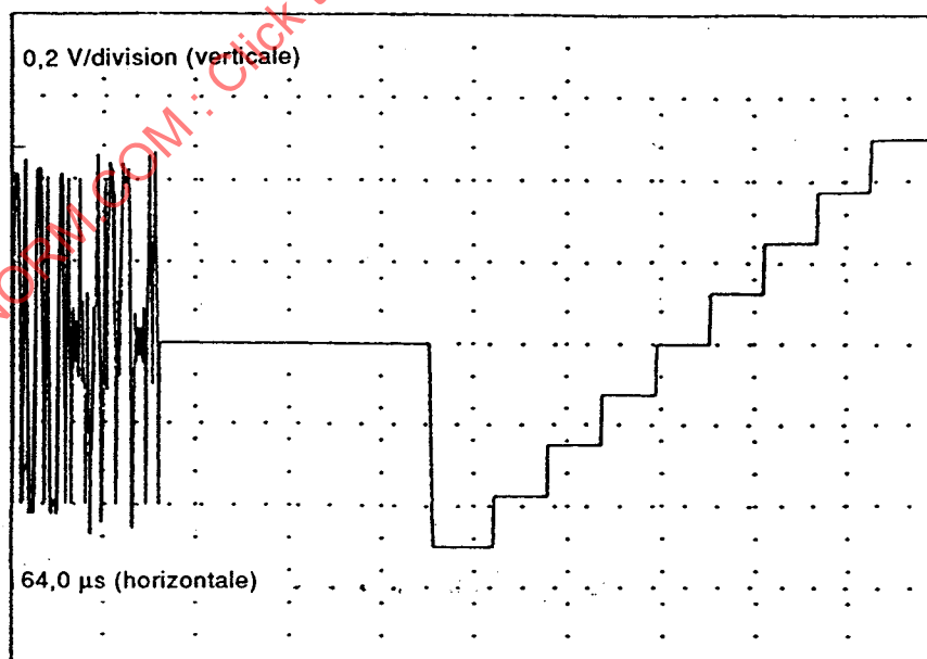
Figure 2g – Signal luminance en escalier à huit fronts montants
