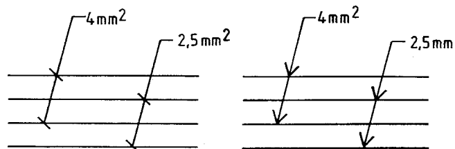
Figure 41 - Lignes de repères aux tracés de connexions
