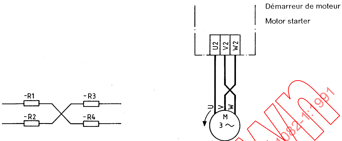
Figure 58 - Exemple de tracés de connexions obliques.
