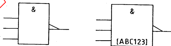
Figure 50 - Exemple de l'utilisation de différentes tailles de symboles; porte -ET avec sortie de complémentarité, sans et avec information supplémentaire.
