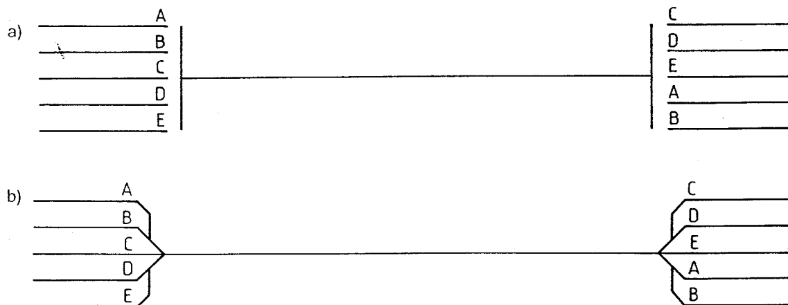
Figure 69 - Exemple de mise en faisceau avec indication des lignes individuelles, méthodes a) et b).
