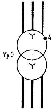
Figure 47 - Exemple d'un symbole complété par les symboles distinctifs pour le raccordement des enroulements et le code de groupe vectoriel; même transformateur que sur la figure 46.
