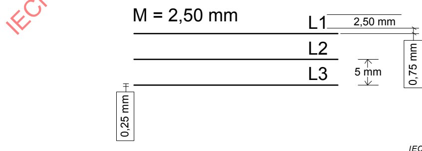
Figure 37 – Espacement des tracés
