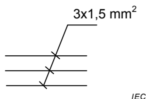
Figure 16 – Exemple d'utilisation de lignes de repère se terminant sur des lignes de connexion
