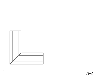
Figure 107c – Disposition pour l'angle extérieur
